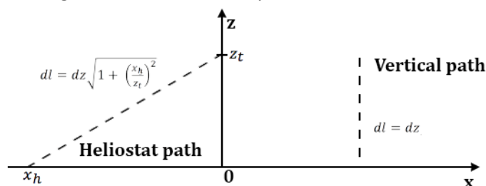
Figura 29 - Descripción del recorrido de la energía entre el heliostato y la torre
