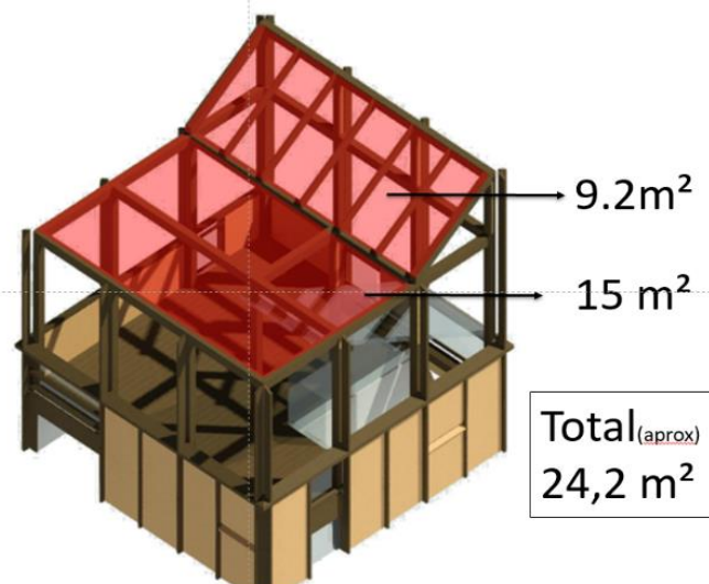
Figura 17 - Configuración de módulos PV
