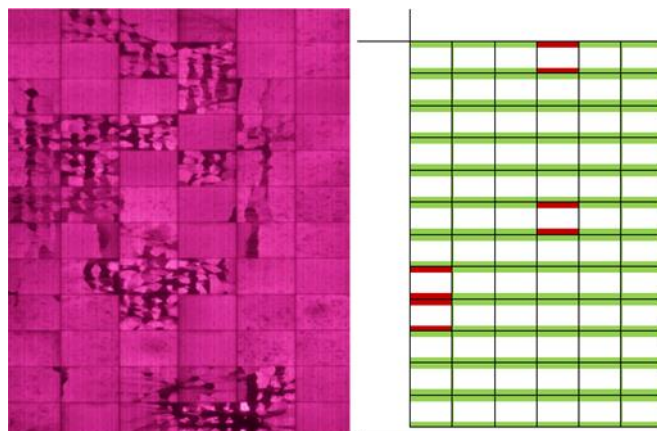
Figura 28 - Módulo PV y su matriz de análisis de celdas dañadas
