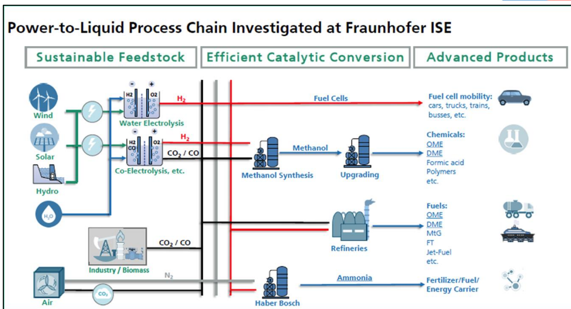
Figura 42 - Cadena Power-to-Liquid, investigada en ISE
